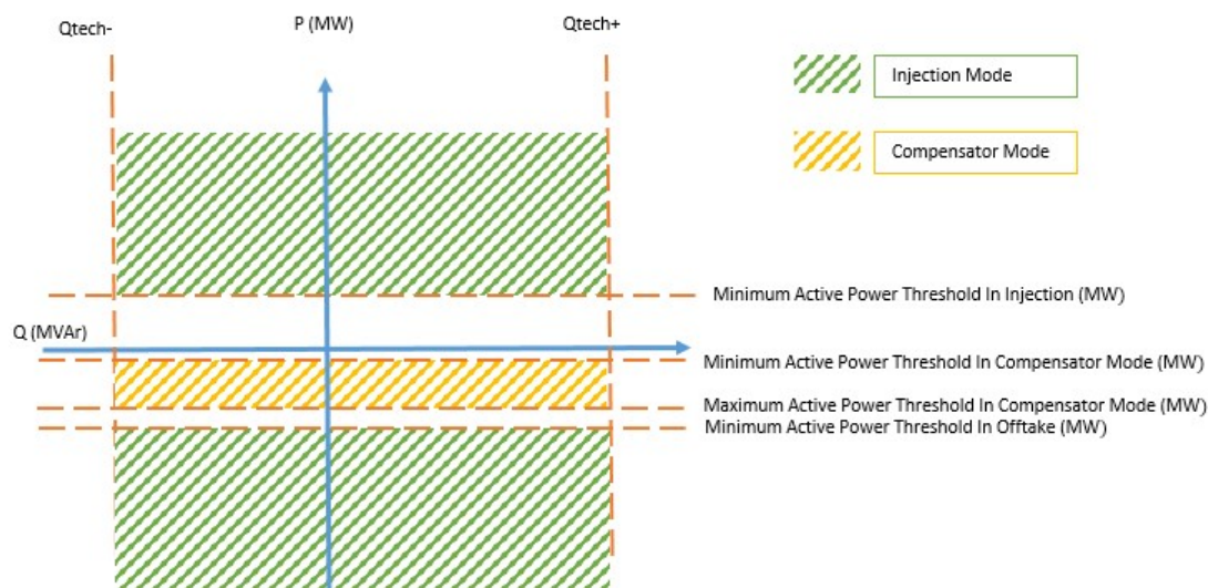
Figure 8 : Unité Technique capable de fournir les Services en Mode injection en injectant ou prélevant de l'Energie Active (option a(i) et a(ii)) et capable de fournir les Services en Mode Compensateur (option b)
