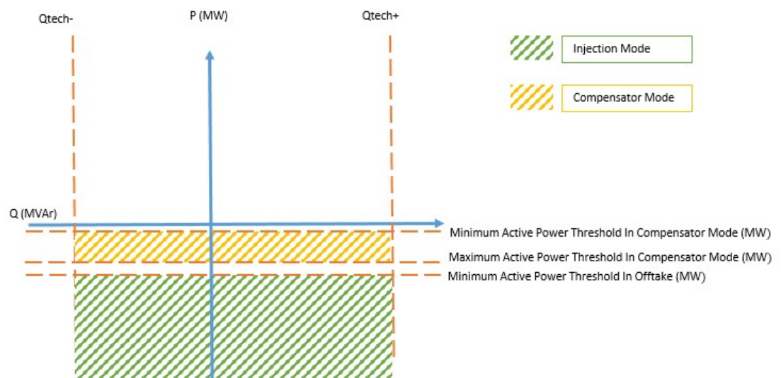
Figure 7 : Unité Technique capable de fournir les Services en Mode injection en prélevant de l'Energie Active (option a(ii)) seulement et capable de fournir les Services en Mode Compensateur (option b)
