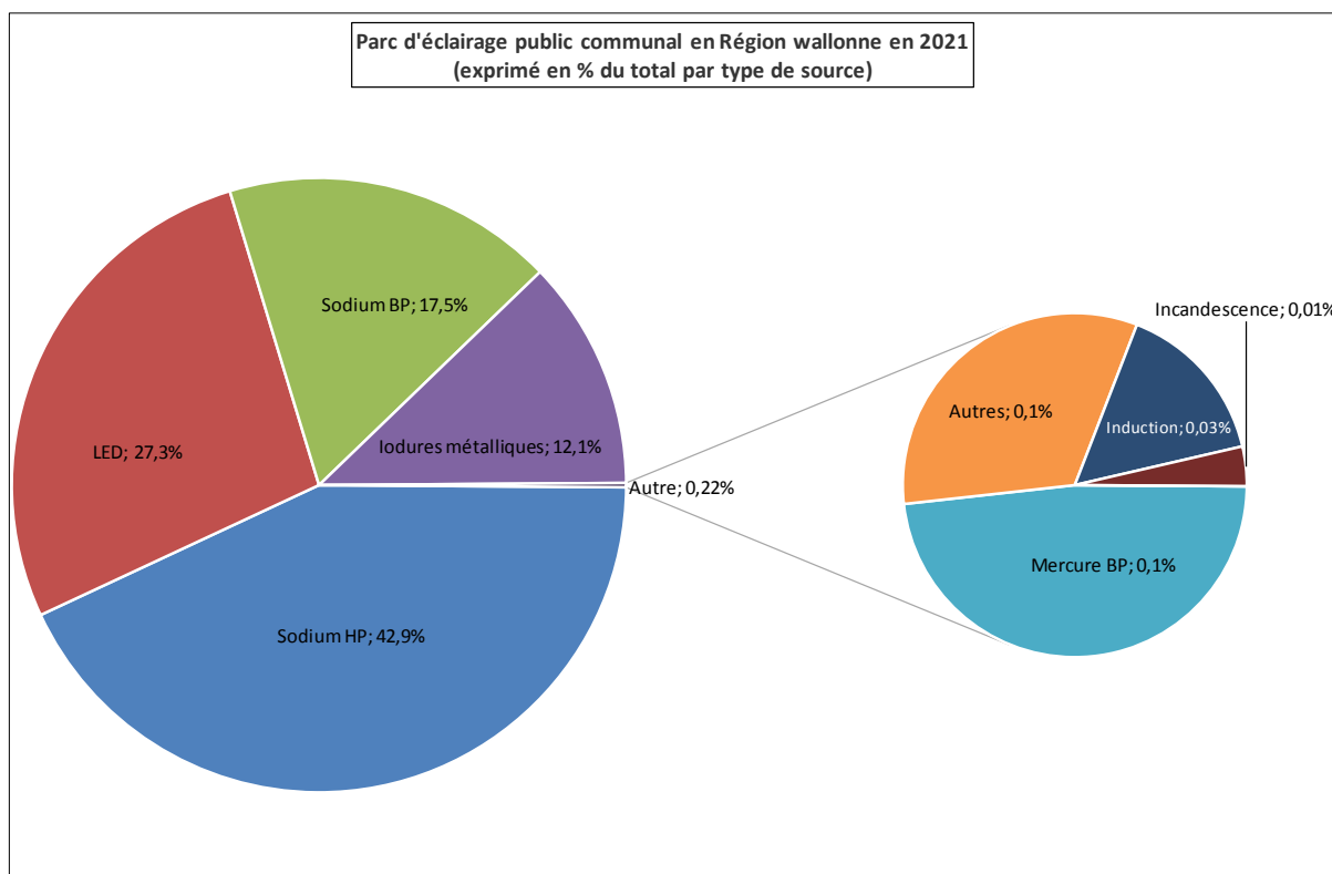
Figure 1 : Inventaire, par type de source lumineuse, à la fin de l'année 2021, pour l'éclairage public fonctionnel et décoratif
