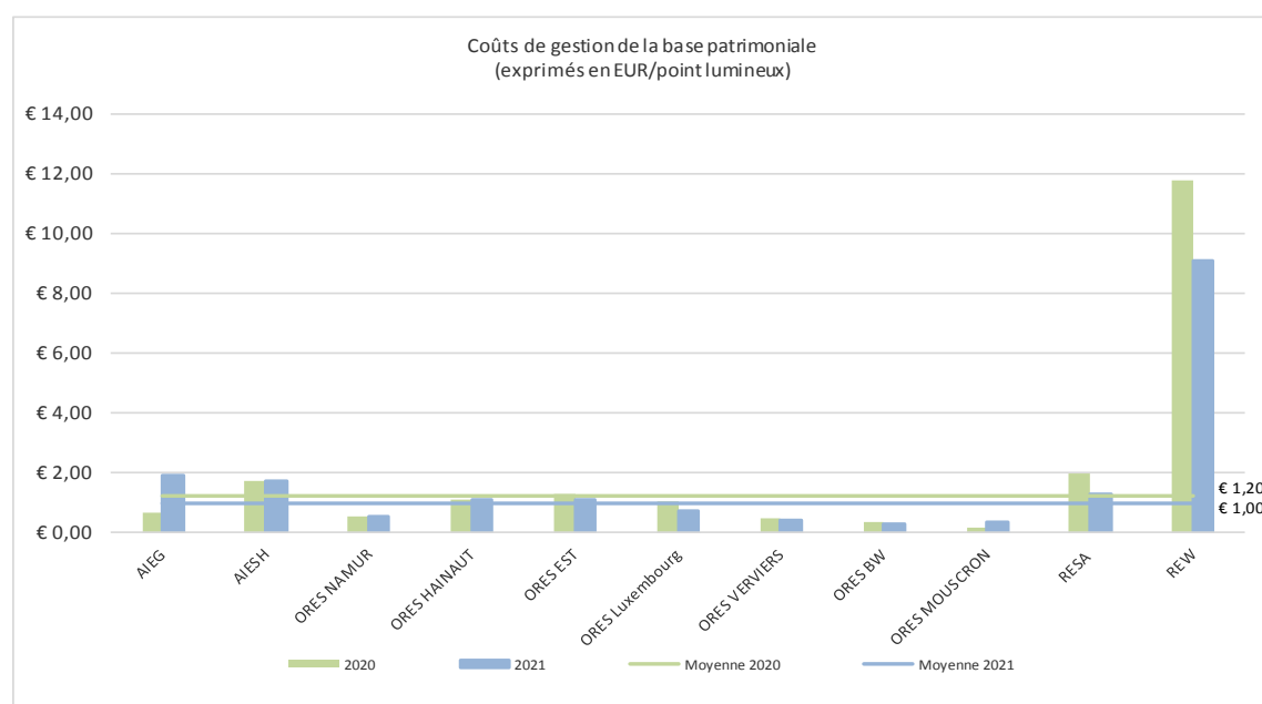
Figure 6 : Évolution des coûts de gestion de la base patrimoniale (EUR/point lumineux)
