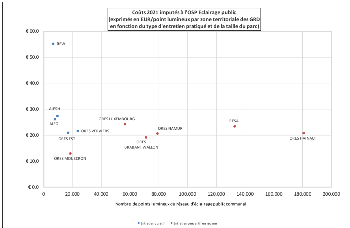
Figure 14 : Coûts 2021 imputés à l'OSP éclairage public (EUR/point lumineux)
