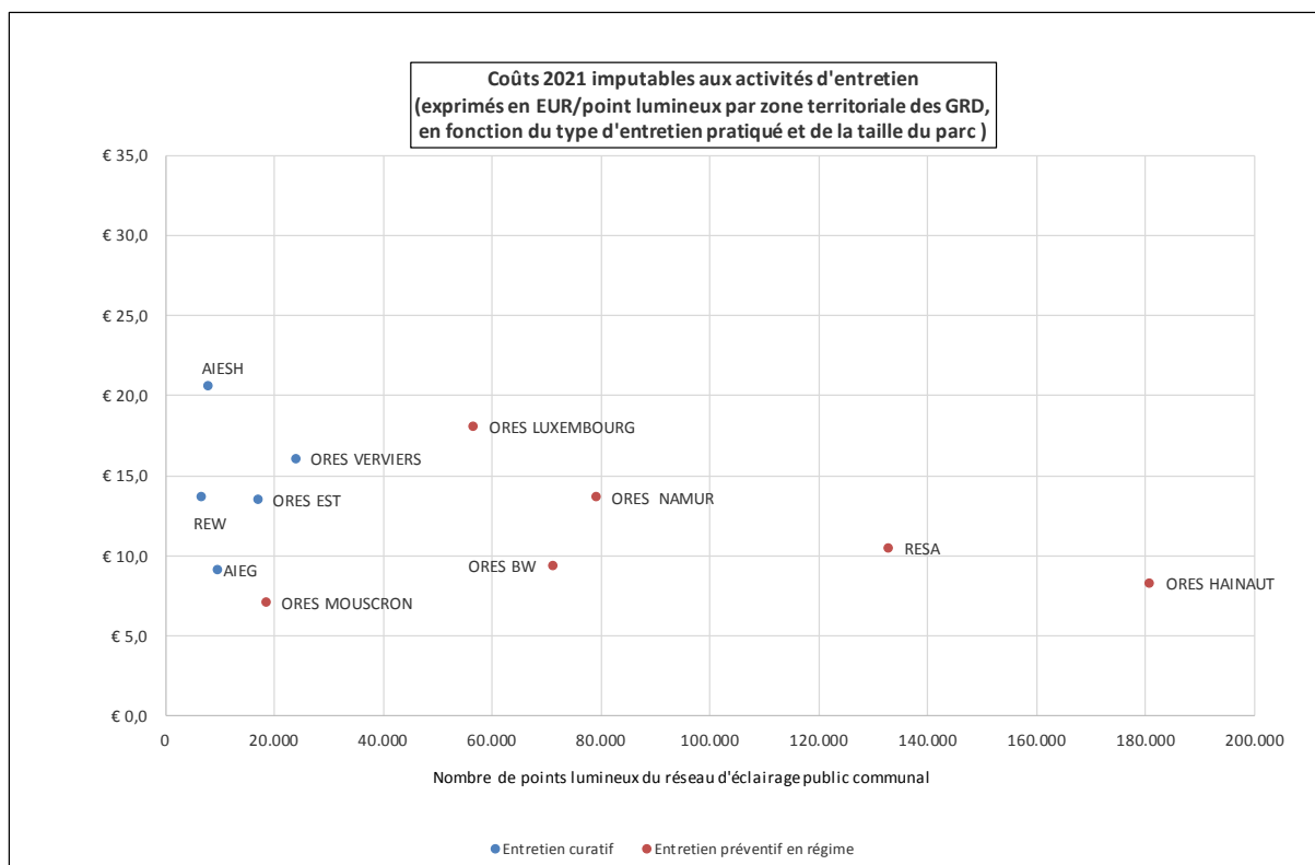
Figure 7 : Coûts 2021 imputables aux activités d'entretien (EUR/point lumineux en fonction du type d'entretien pratiqué et de la taille du parc)
