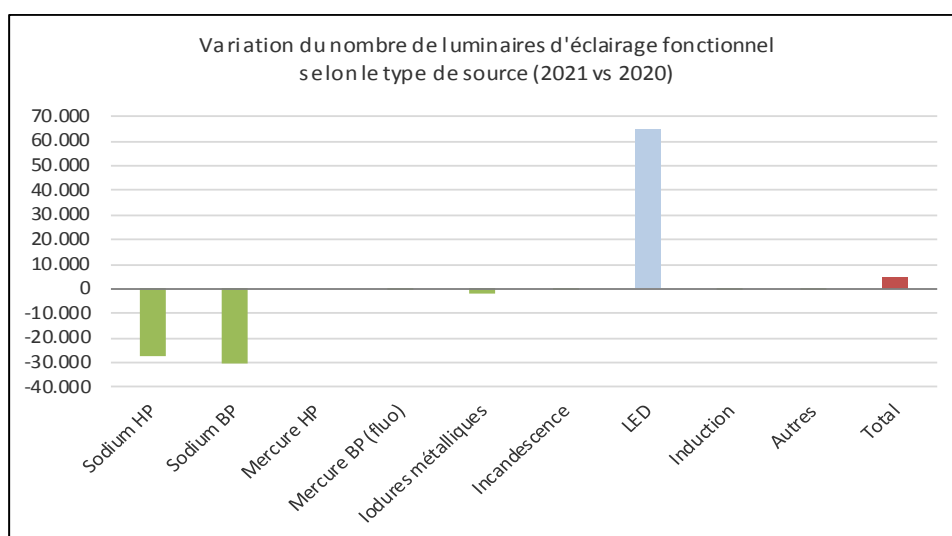
Figure 3 : Variation du nombre de luminaires d'éclairage public fonctionnel selon le type de source
