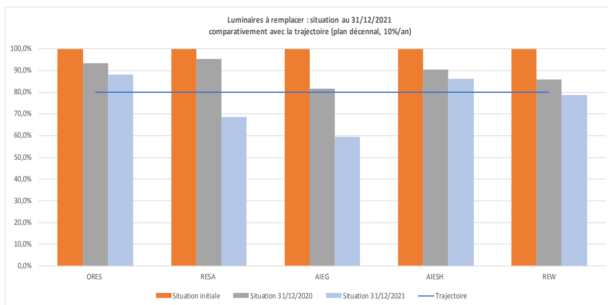
Figure 10 : Situation du plan de remplacement décennal au 31/12/2020 comparativement à la trajectoire
