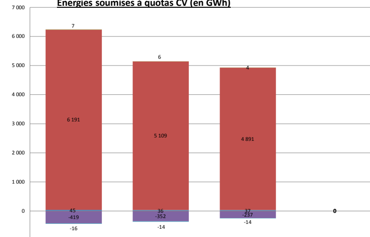
Energies soumises à quotas CV (en GWh)
